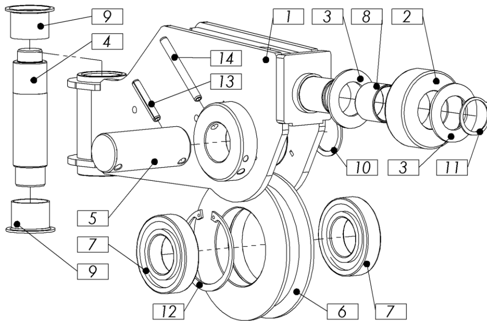
Bild 13: 801.25.70.A – Seilverteiler kpl.
