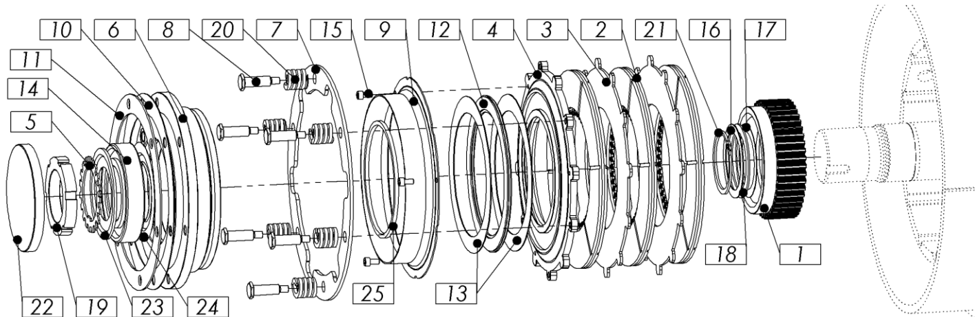
Bild 6: 801.03.00.0 – komplett
