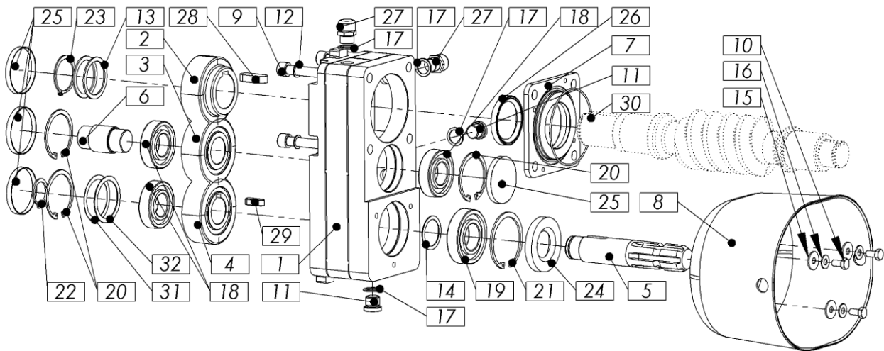
Bild 3: 801.01.80.0 - Eingangsgetriebe
