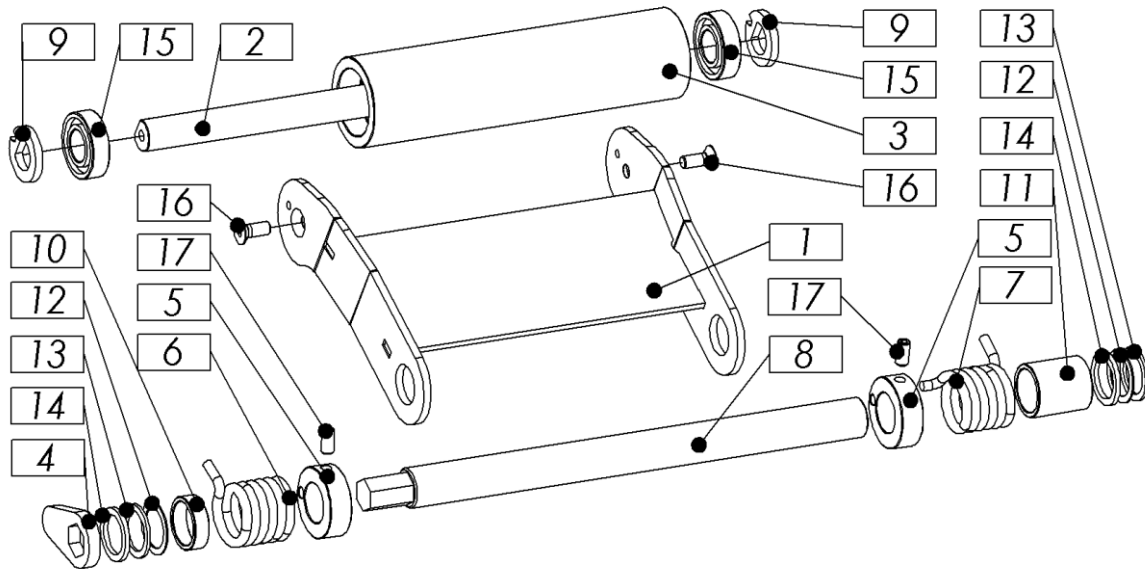
Bild 4: 801.01.100.0 – Rolle kpl.
