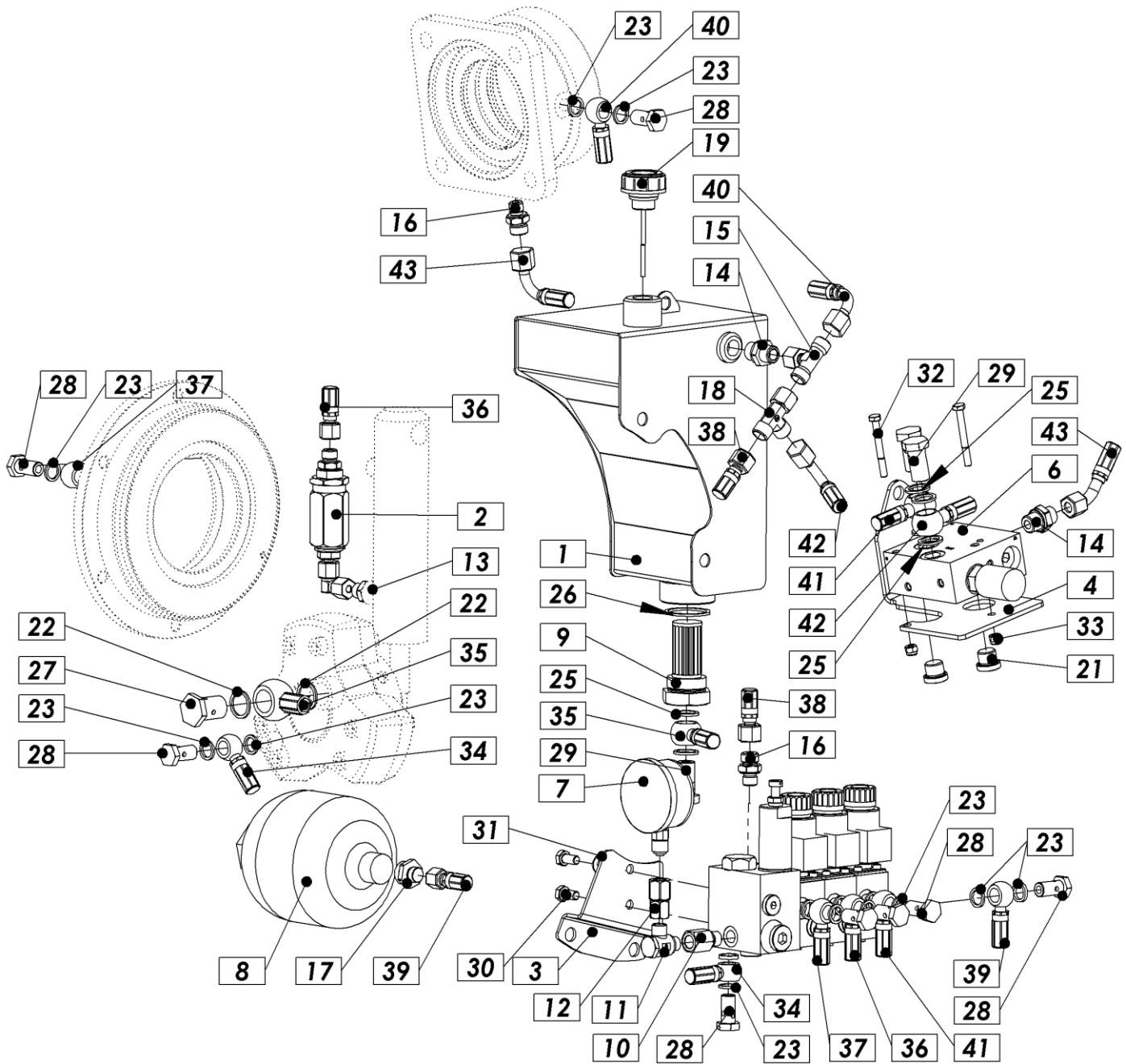
Bild 10: 801.06.00.0 – Hydraulikaggregat
