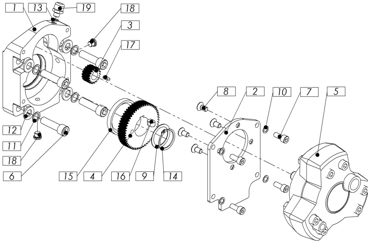
Bild 2: 801.01.60.0 – Untersetzung komplett
