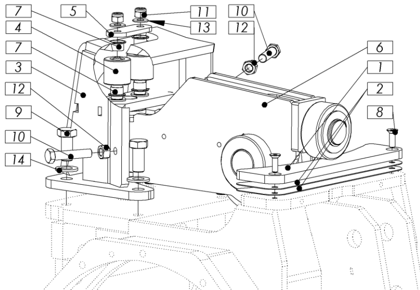
Bild 14: 801.25.200.0 – Aufwicklung komplett.
