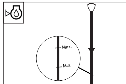
Abb. 5.3a Ölmessstab-Markierungen
