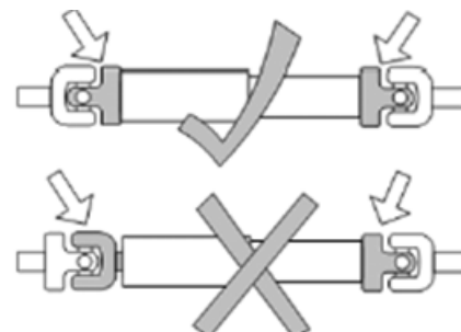
Gabeln korrekt ausrichten 1 - Z-förmige Gestaltung 2 - W-förmige Gestaltung
