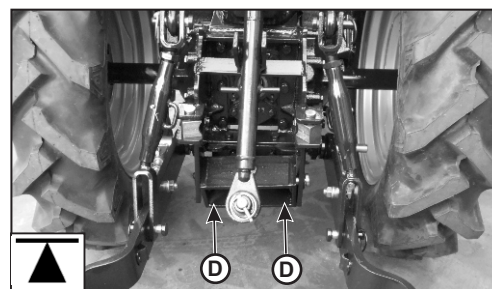
Abb. 5.23b - Traktorrhinseite anheben
