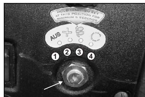
Abb. 4.3.1a - Startschalter für Modell 20
