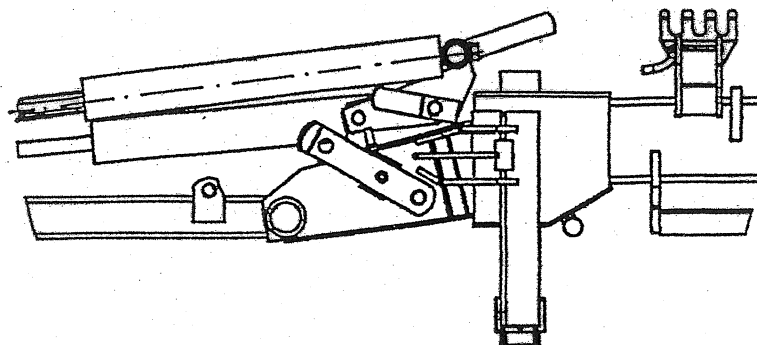
Bild 7 Fig. 7 Arbeitsstellung des Mähers Mower's working position
