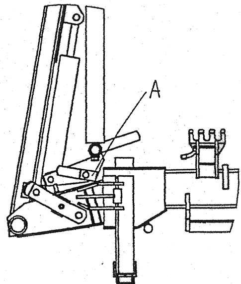
Bild 6 B Fig. 6 B Fixierung der Entlastungsfedern (Mähebalken in senkrechte position) Fixation of relieve springs by a pin (Cutter bar in upright position)
