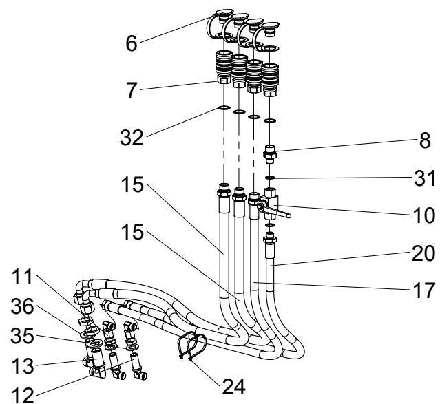
Bucher Letran
