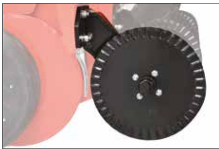
Vordere Schneidscheibe ø 355 mm
