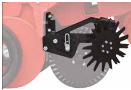
Räumstern ø 355 mm zur Schneidscheibe (nicht geeignet für Geräte mit Düngerscharen)
