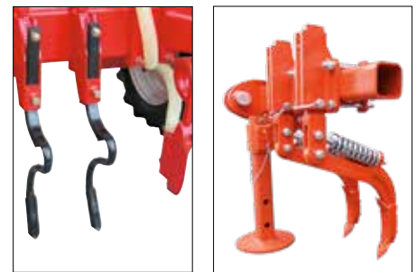
Satz Spurlockerer (4 Stück), starr für MTR, gefedert für MIRKA-MANTA
