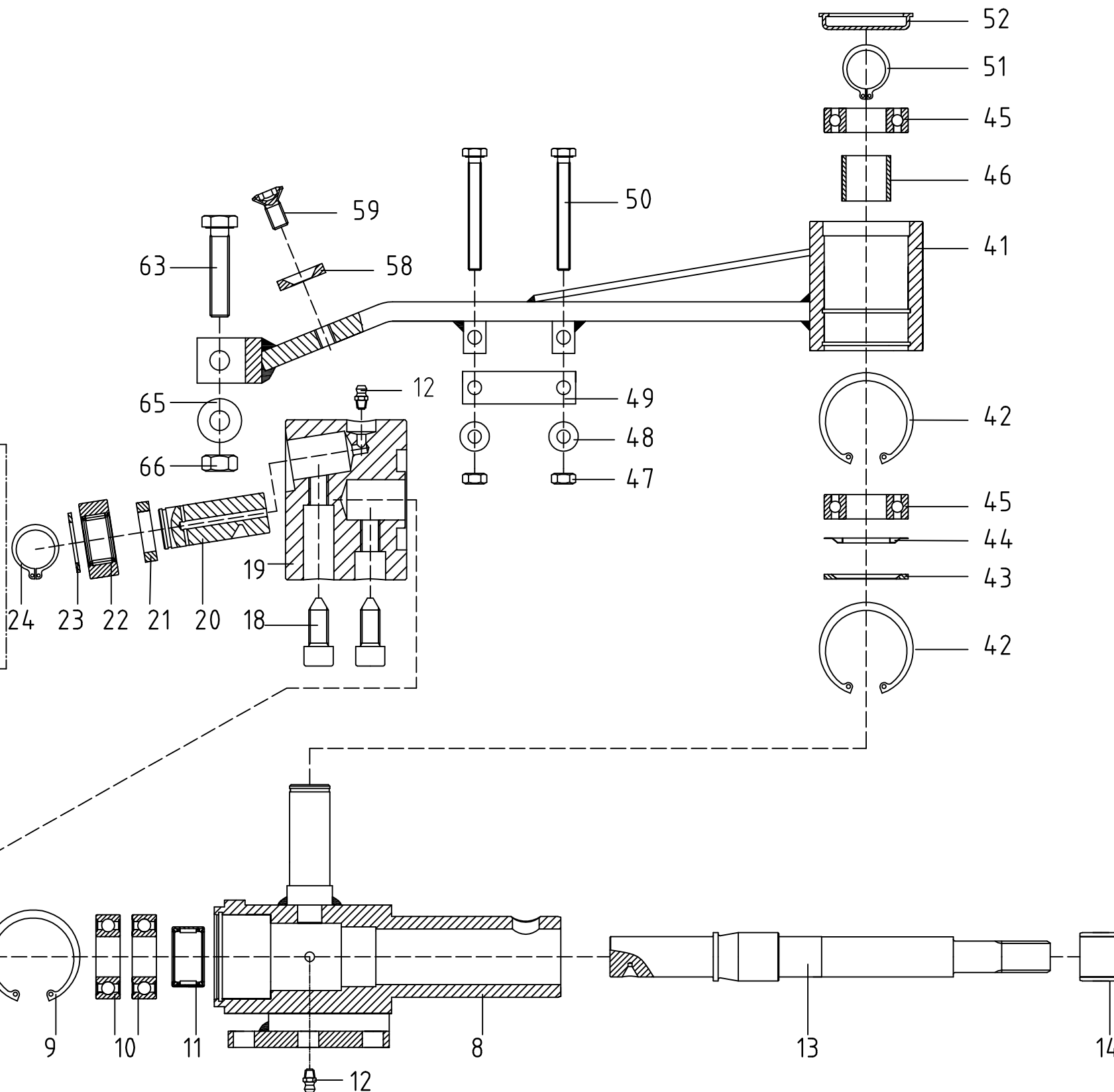
Schnitt A-A
